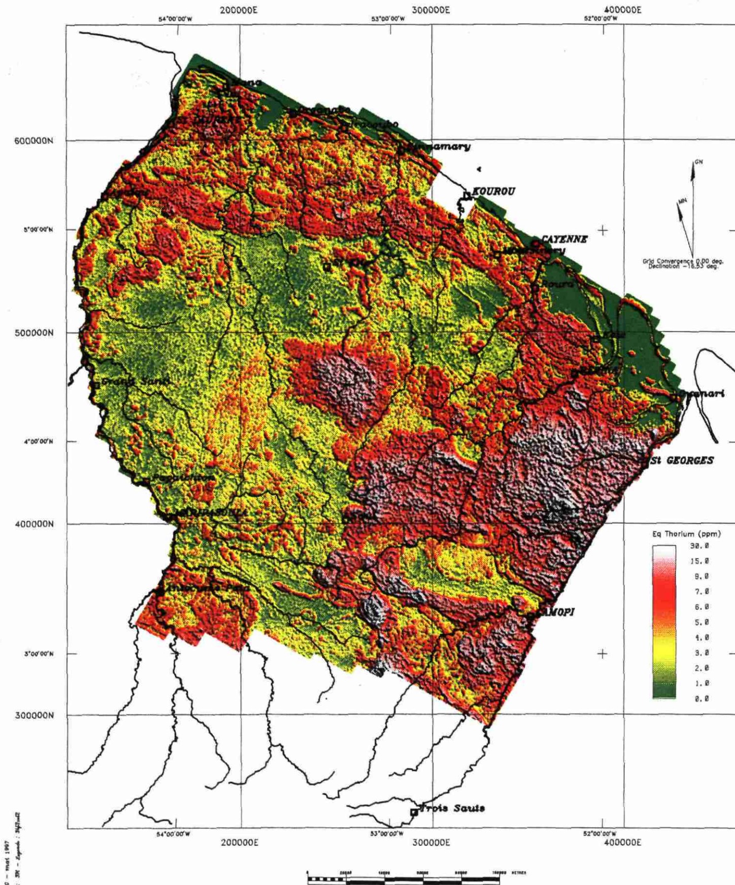
Fig. I - Radiométrie spectrale - Thorium.
