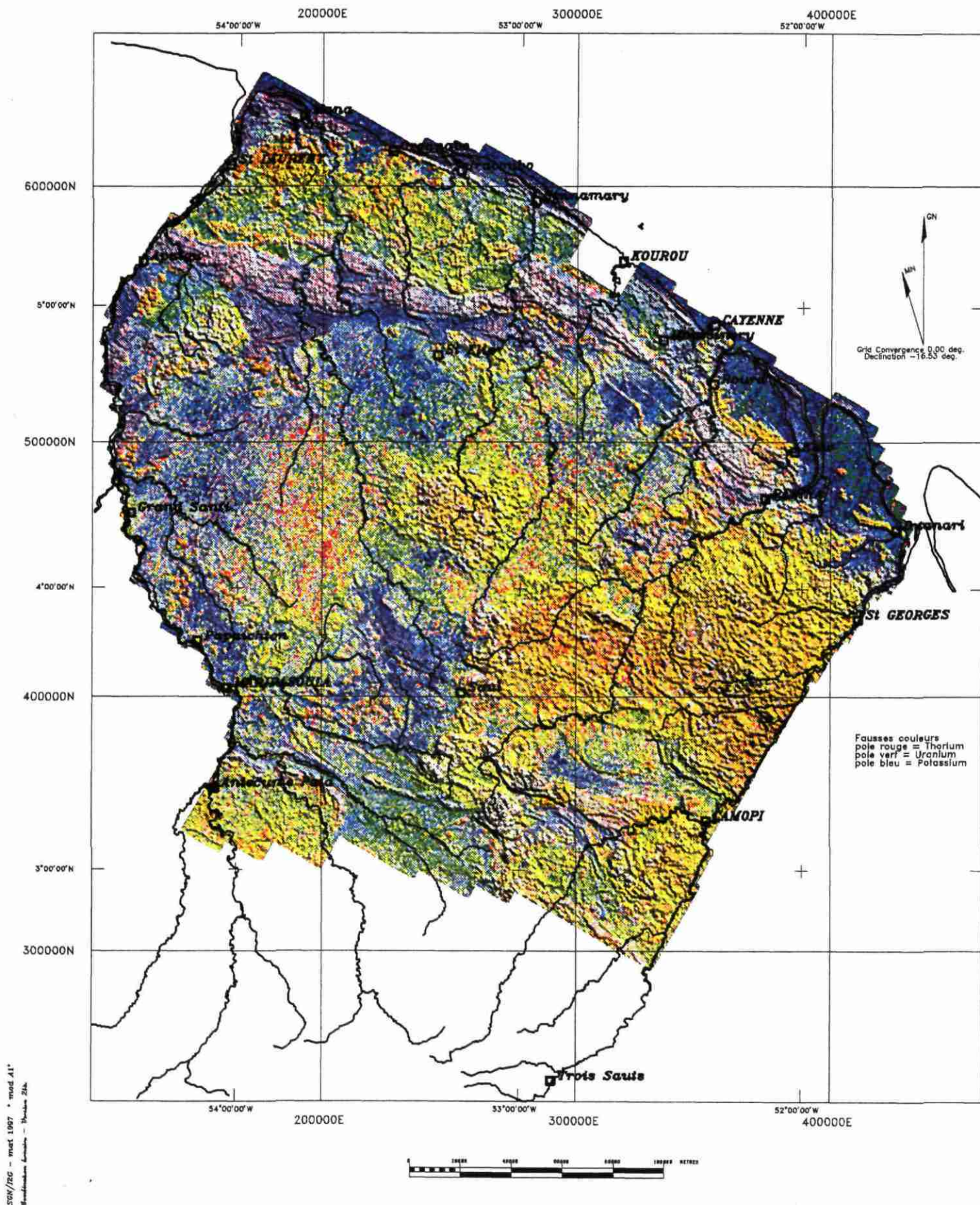
Fig. K - Radiométrie spectrale - Combinaison ternaire Th/U/K.
